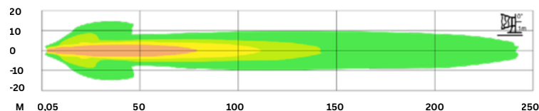
isolux E-DHL-90, Low beam, H.:1.0m, tilt: 0°,1lux@140+m
