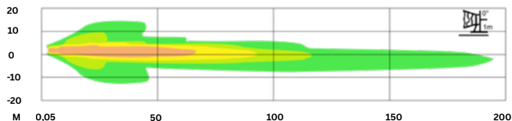
isolux E-DHL-90, Low beam, H.:1.0m, tilt: 0°,1lux@140+m
